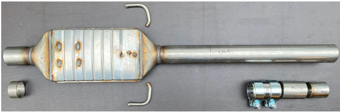
Leveringsomfang. Kombifilter DPF-06, katalysator+DPF, med Ø60/Ø56mm rustfri rør, plus rustfri fittings
